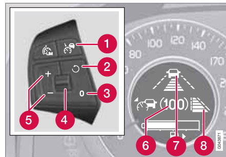
Commandes au volant 3 et écran.
