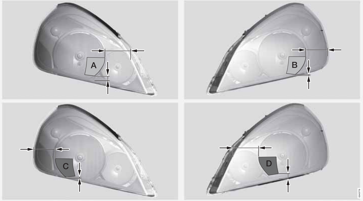
Ligne supérieure : masquage pour voiture avec conduite à gauche, modèles A et B. Ligne inférieure : masquage pour voiture avec conduite à droite, modèles C et D.
